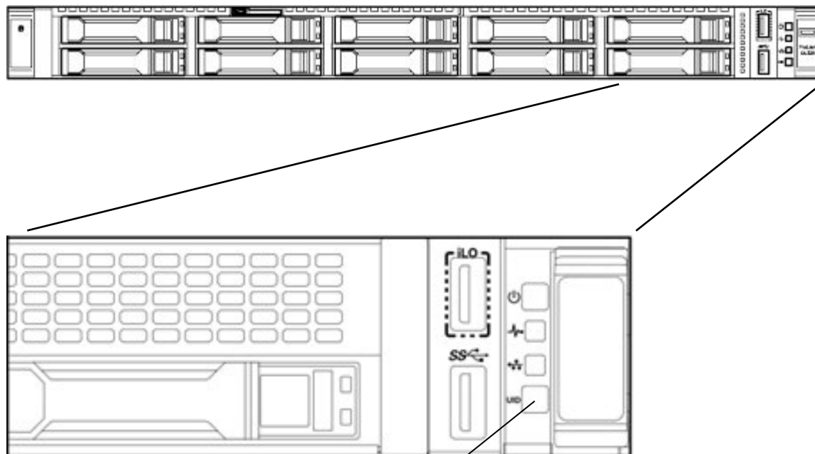
前面 8x2.5 型ドライブモデル
