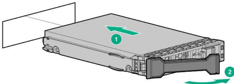
2.5 型ドライブ
