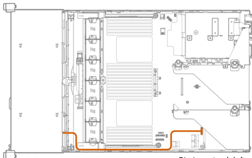
Displayport コネクタ
