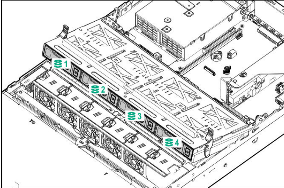
3.5 型ドライブモデルのミドルドライブケージ 4x3.5 (SAS/SATA HDD)
