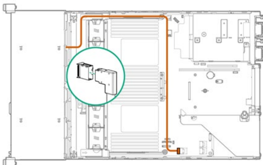
② SAS/SATA ドライブケージ (N8154-96) 、RAID コントローラーに接続の場合
