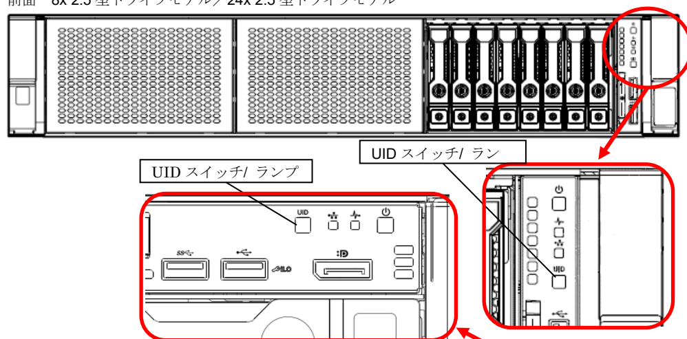
前面 8x 3.5 型ドライブモデル
