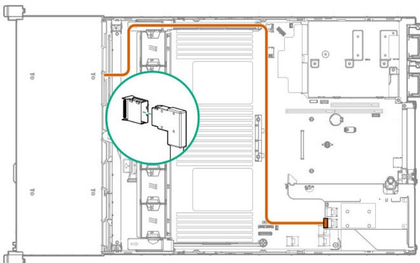
③ SAS/SATA ドライブケージ (N8154-96) 、SAS エキスパンダに接続の場合
