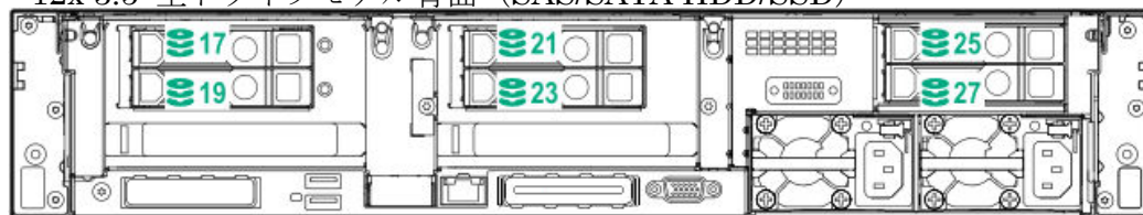
12x 3.5 型ドライブモデル背面 (SAS/SATA HDD/SSD)
