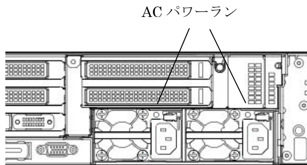
電源ユニット
