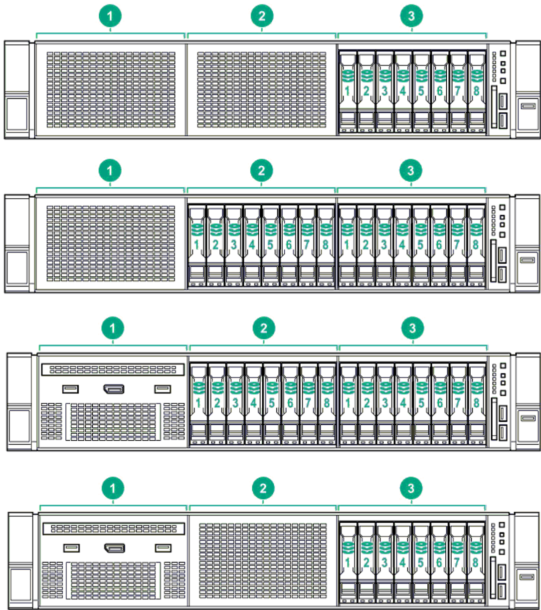
2.5 型ドライブモデル フロント BOX
