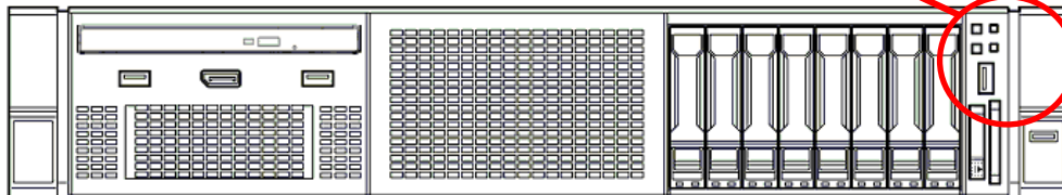
前面 8x 2.5 型ドライブモデル ステータス LED パネル (オプション)
