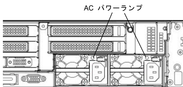
電源ユニット 2 電源ユニット 1
