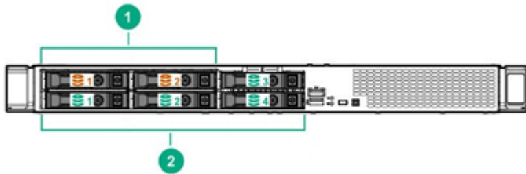
4x2.5 型ドライブモデル+2 x 2.5 型 HDD/SSD(オプション)
