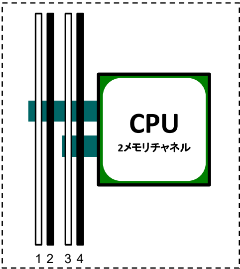
サーバ本体前面側
