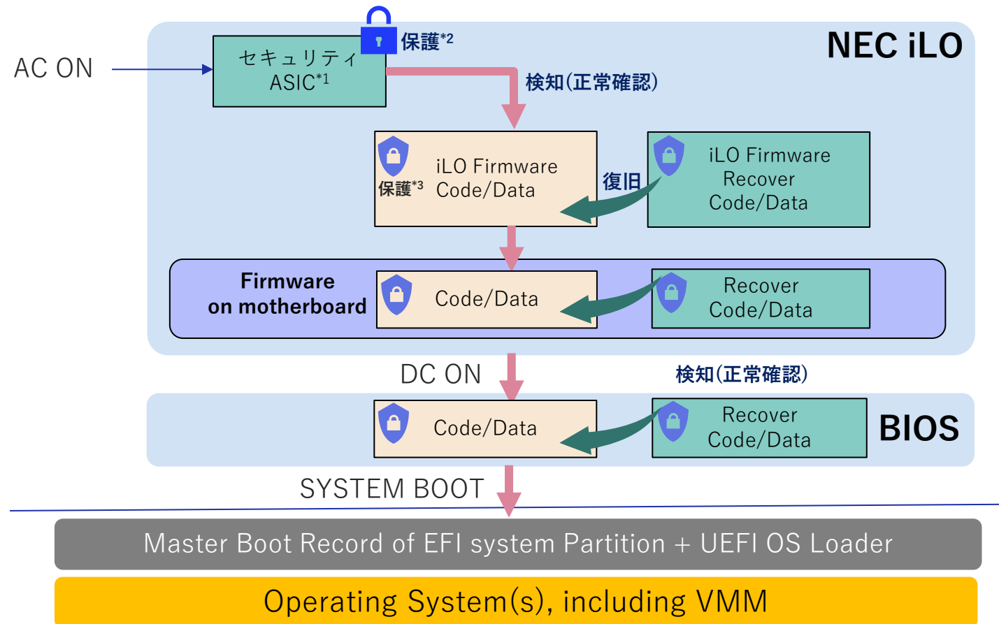
Fig.2 NEC Express5800 / NX7700xシリーズのNIST SP 800-193の取り組み
