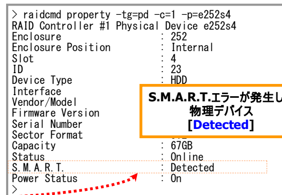
図 30 RAID ビューア/raidcmd の表示(S.M.A.R.T.エラー検出)
